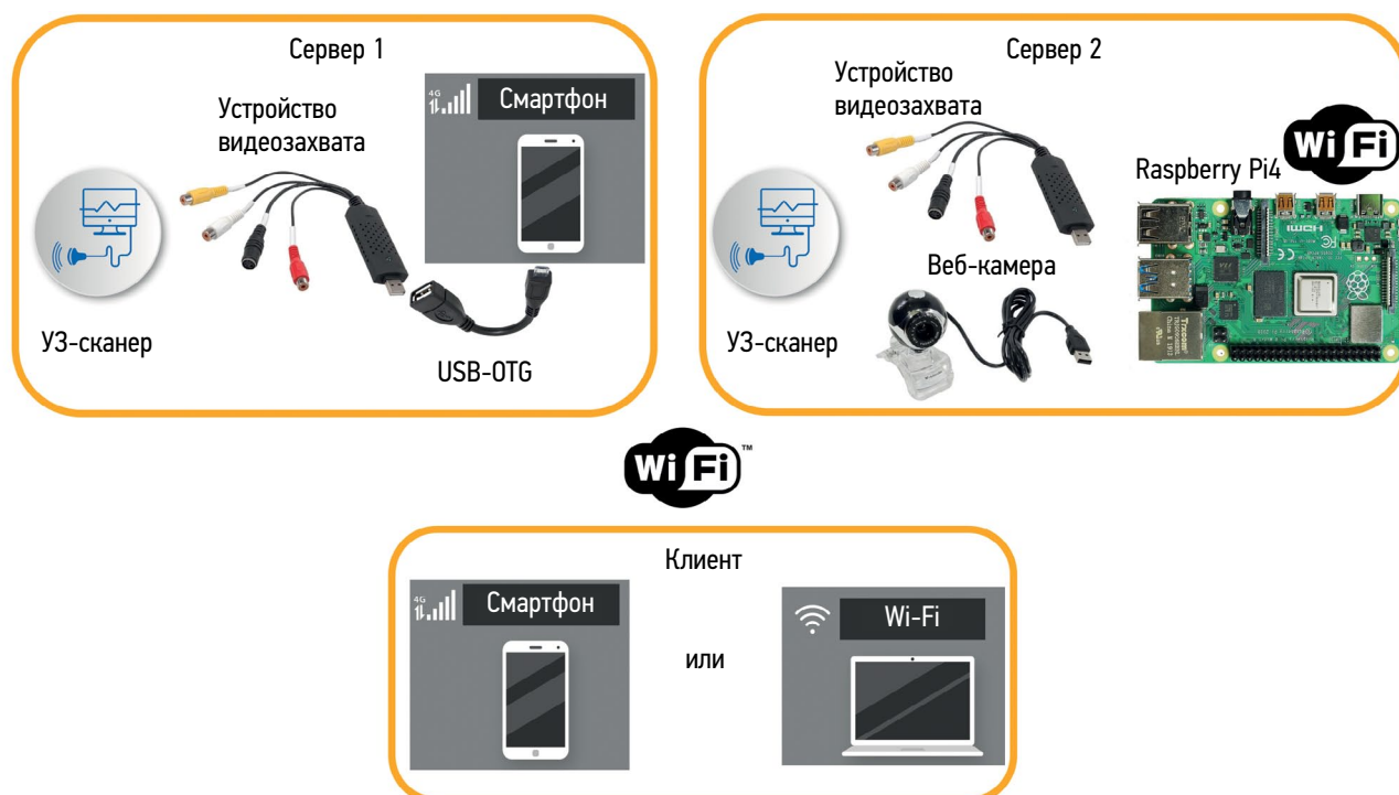
Рис. 1. Схема подключения.
